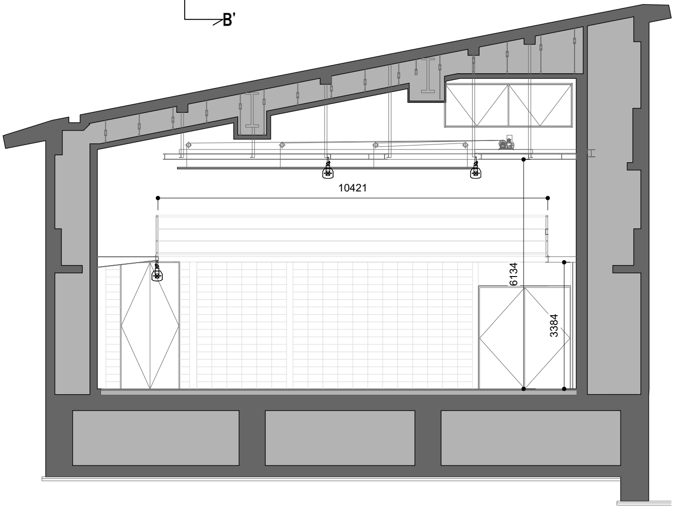
A-A' 断面図
