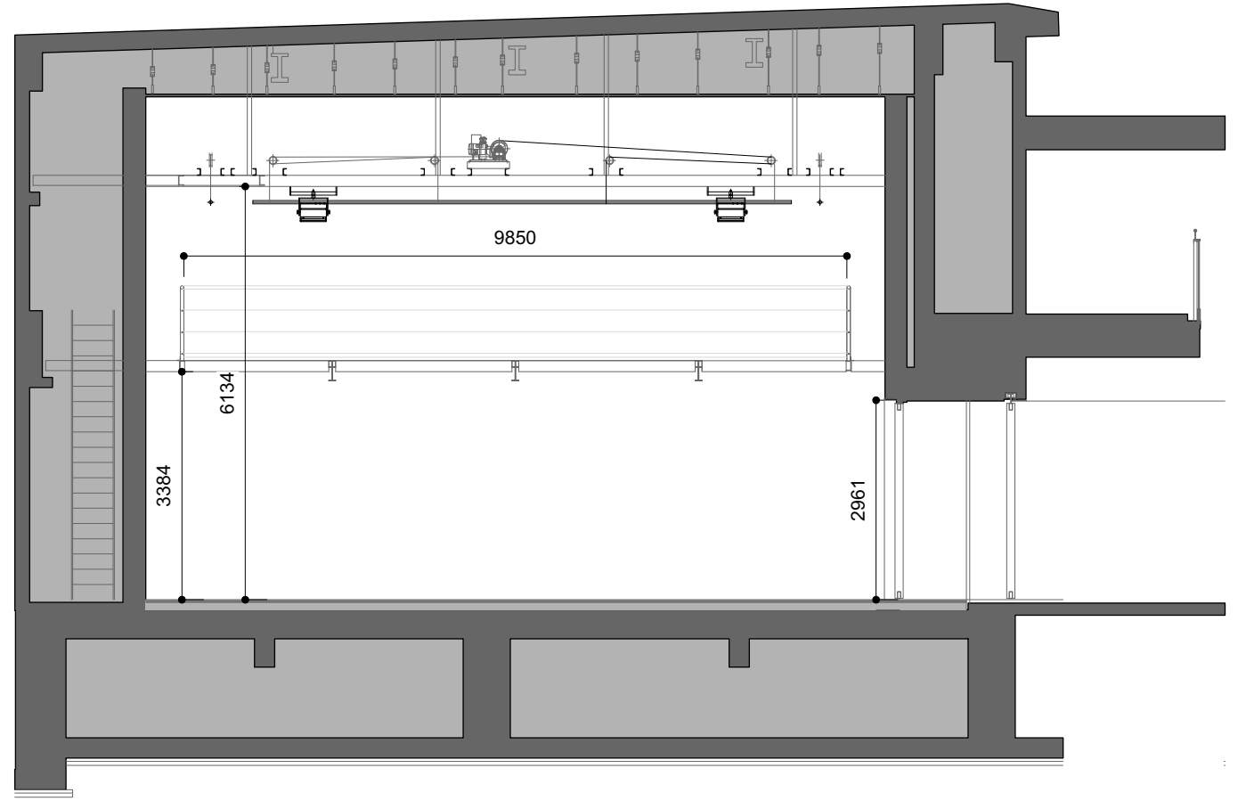
B-B' 断面図
